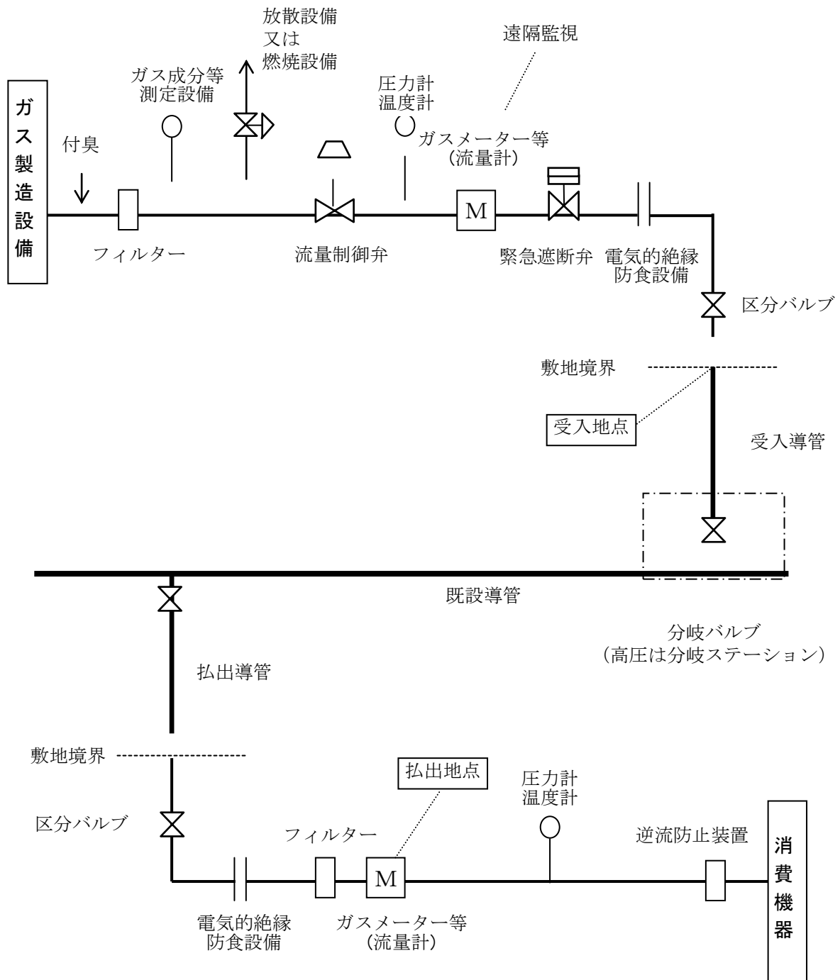
(参考) ガスの受入及び払出のために必要となる設備概要 (概念図)
